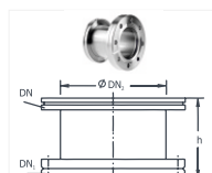
Адаптеры ISO-K / CF
